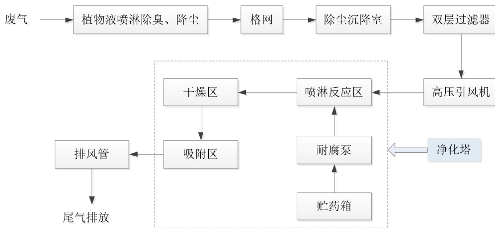
图 8 植物液喷淋+负压抽风除尘除臭系统工艺流程图
